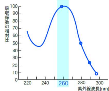
■ 細菌のDNAの分光特性
