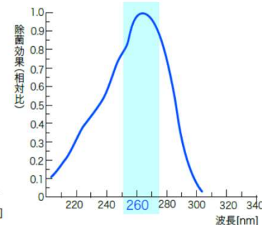
■ 除菌作用の分光特性
